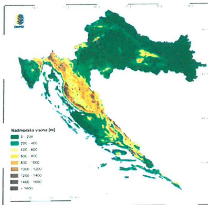
Slika 15. Topografija Hrvatske s mrežom mjernih postaja
