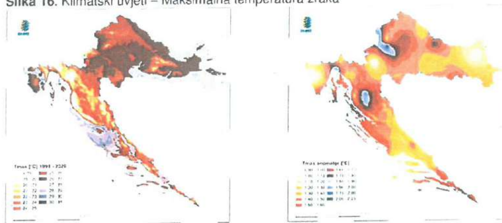
Slika 16. Klimatski uvjeti – Maksimalna temperatura zraka
