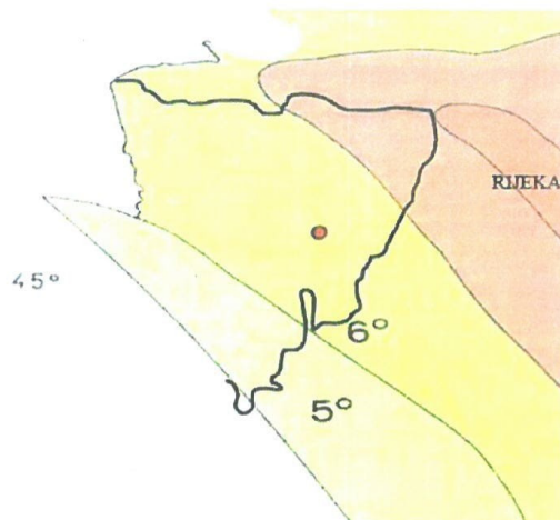
Slika 5. Seizmološka karta za povratni period od 50 godina
