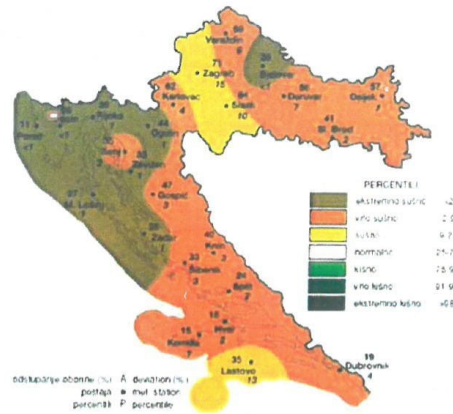
Slika 31. Odstupanje količine oborine za ljeto
