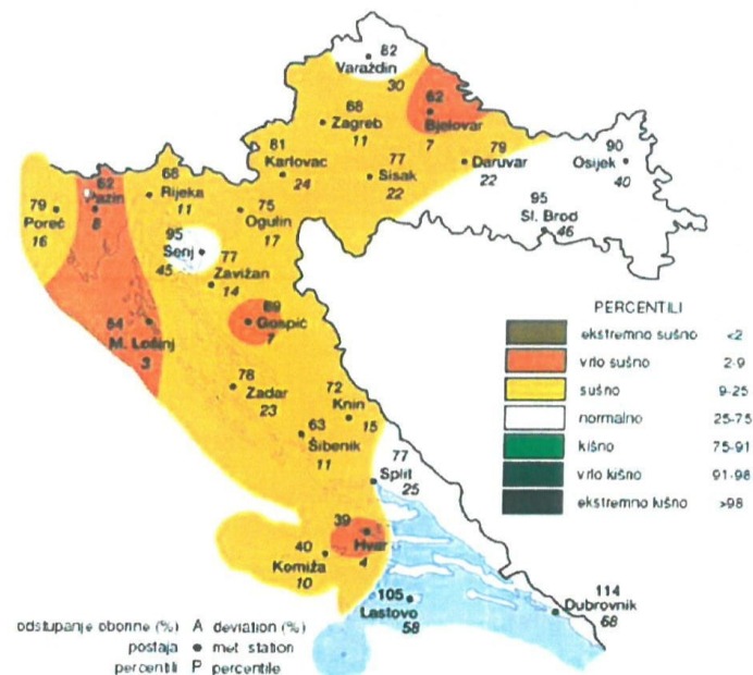
Slika 30. Odstupanje količine oborine za proljeće
