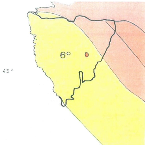
Slika 7. Seizmološka karta za povratni period od 200 godina Izvor: V. Kuk, PMF Zagreb, Geofizički odsjek
