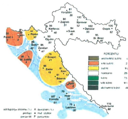
Slika 32. Odstupanje količine oborine za zimu
