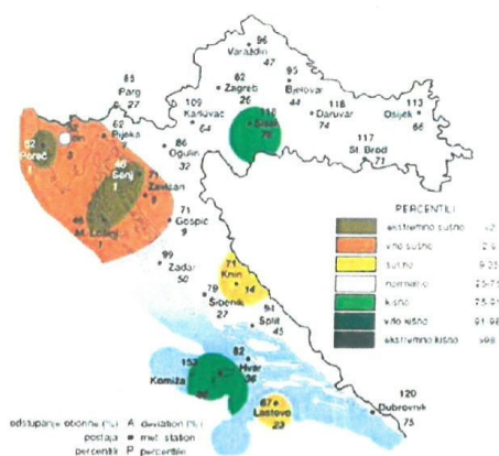
Slika 33. Odstupanje količine oborine za jesen Izvor: DHMZ
