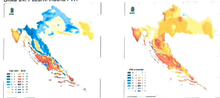
Rast FWI gotovo u cijeloj zemlji tijekom požarne sezone Izvor: Državni hidrometeorološki zavod 2023.
