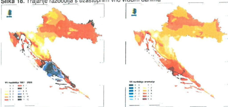
Slika 18. Trajanje razdoblja s uzastopnim vrlo vrućim danima
