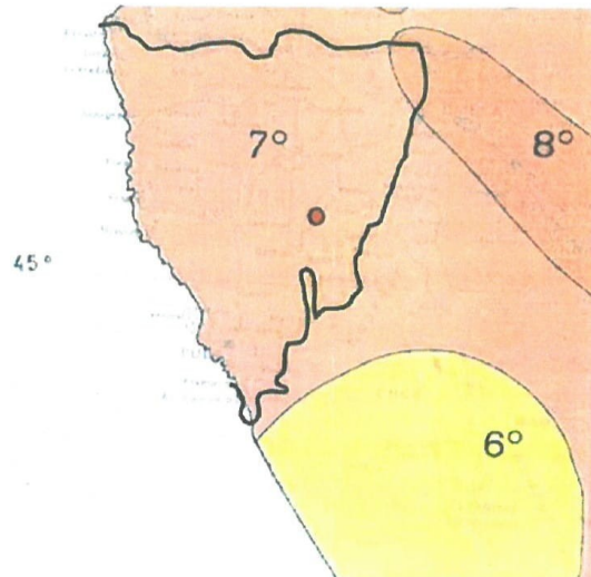
Slika 8. Seizmološka karta za povratni period od 500 godina Izvor: V. Kuk, PMF Zagreb, Geofizički odsjek
