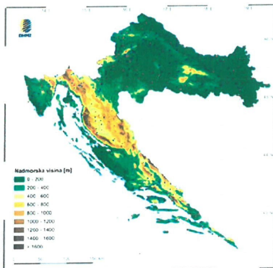
Slika 15. Topografija Hrvatske s mrežom mjernih postaja
