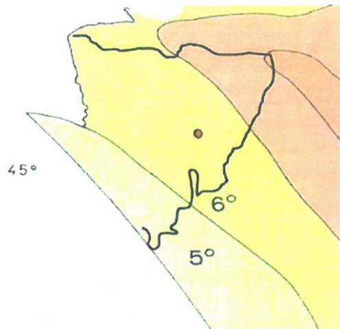
Slika 6. Seizmološka karta za povratni period od 100 godina
