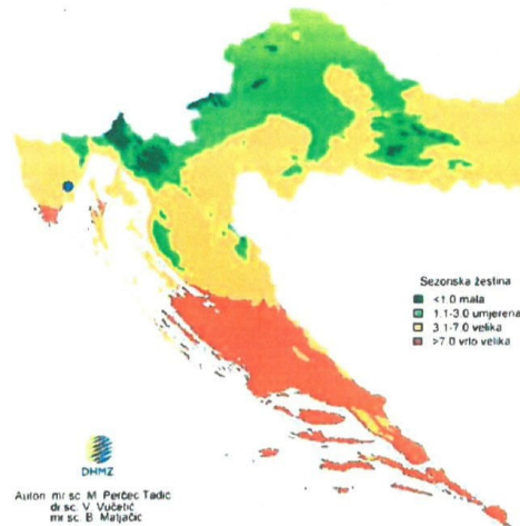
Slika 26. Karta indexa potencijalne opasnosti od požara raslinja u sezoni
